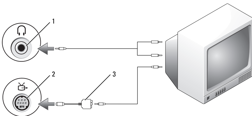
1 connecteur d'entrée audio 2 connecteur de sortie TV S-vidéo 3 adaptateur vidéo composite
