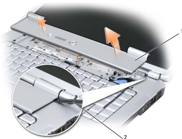
1 cache de charnière 2 pointe
