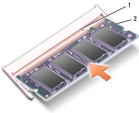
1 languette 2 encoche
