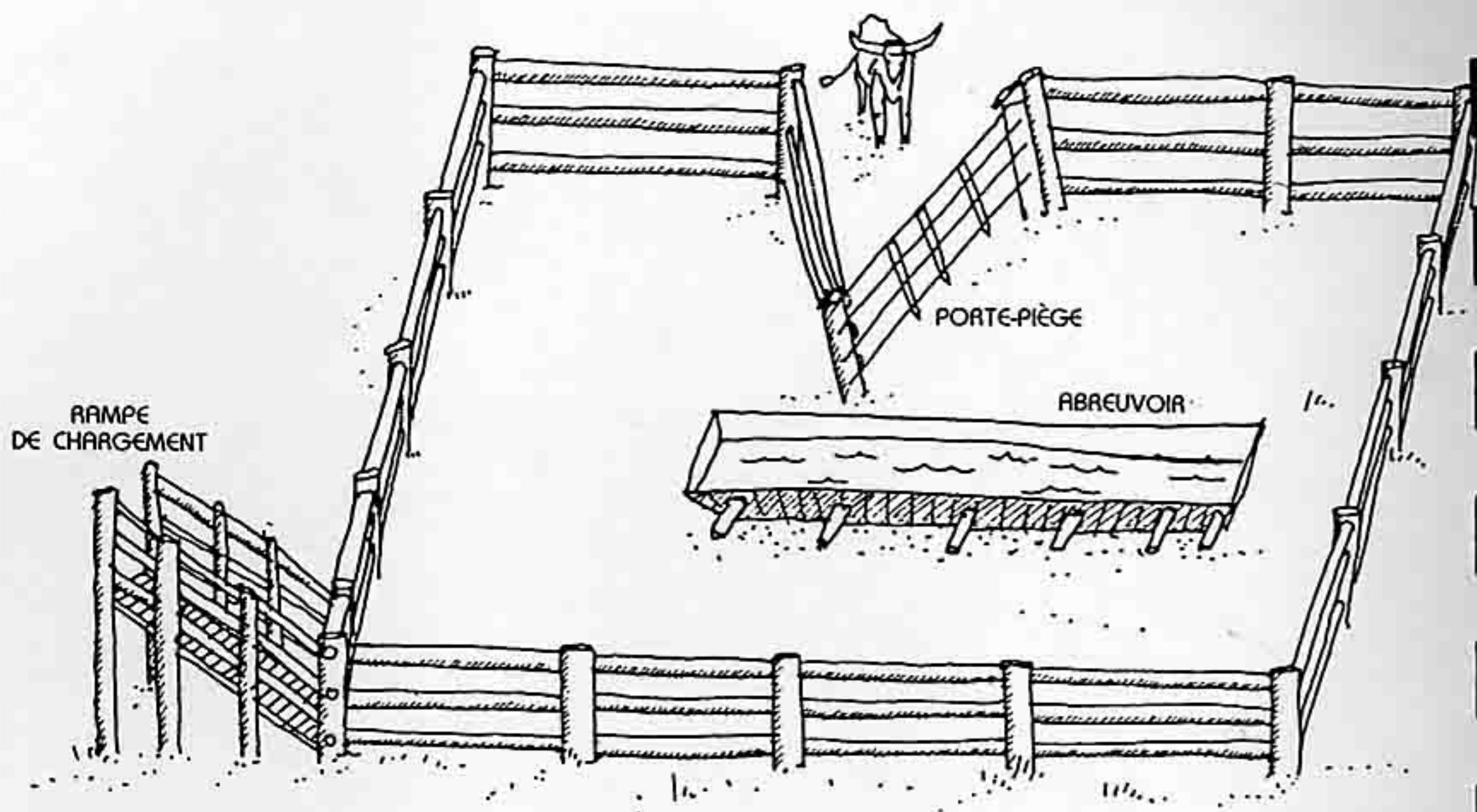
FIG. 5.22 : ENCLOS-PIÈGE. L'ABREUVOIR ATTIRE LES HERBIVORES REDEVENUS SAUVAGES.
