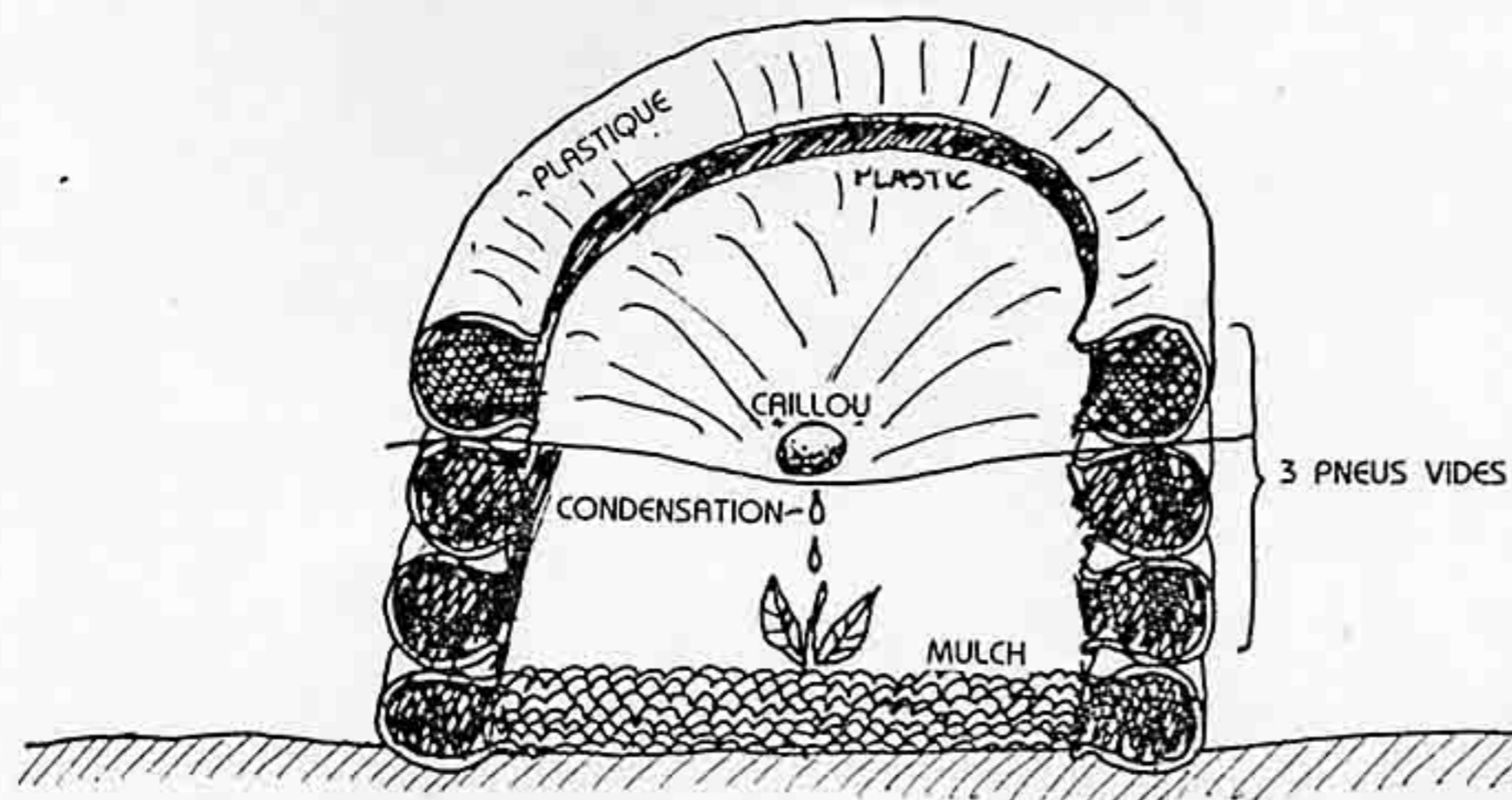
FIG. 5.21 : SERRE EN PNEUS. LE PLASTIQUE CONDENSE L'HUMIDITÉ DE LA NUIT. LA FEUILLE DE PLASTIQUE EST RETIRÉE A LA FIN DU PRINTEMPS. AUTO-ARROSÉ ET RÉSISTANT AU GEL.
