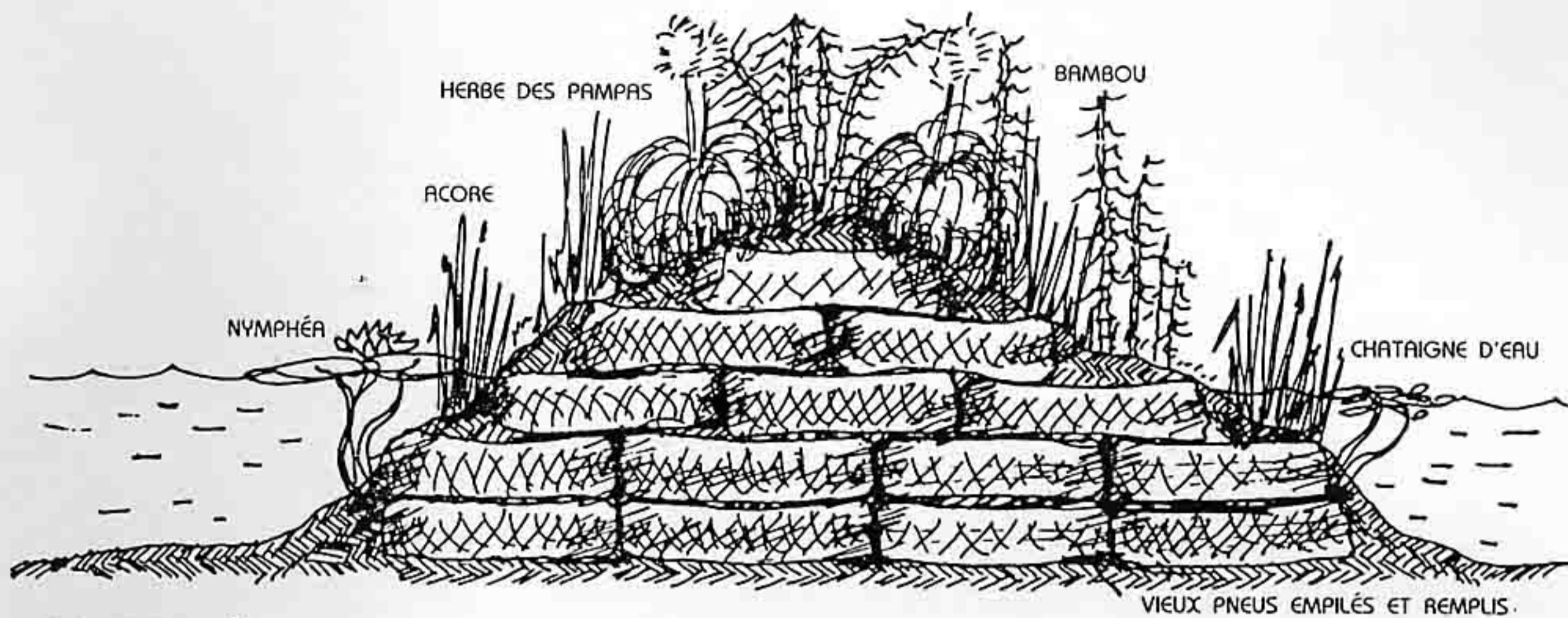
FIG. 7.20 : ÎLE DE PNEUS.
