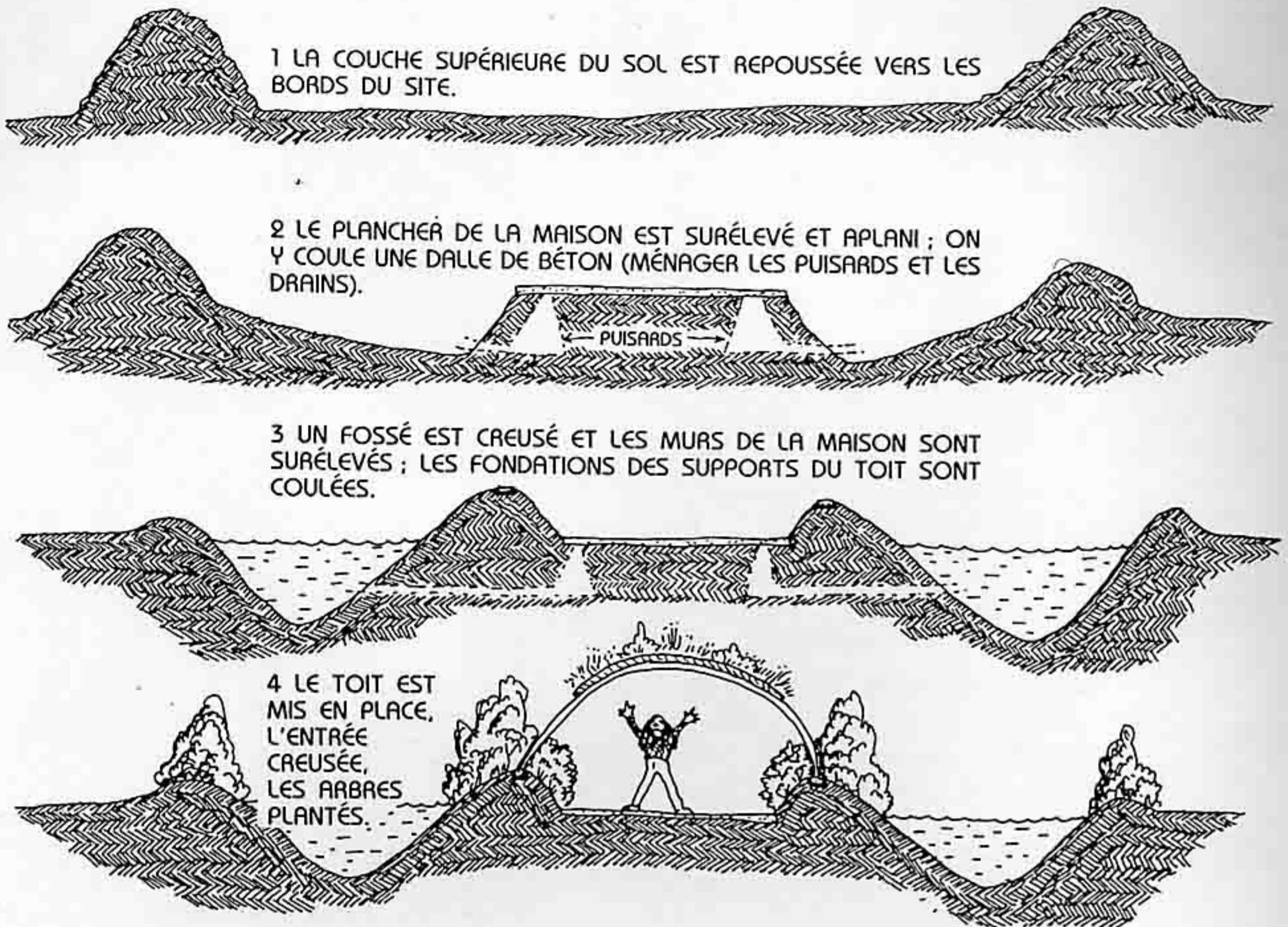
FIG. 6.5 : STADES DE CONSTRUCTION D'UNE MAISON EN TERRE.
