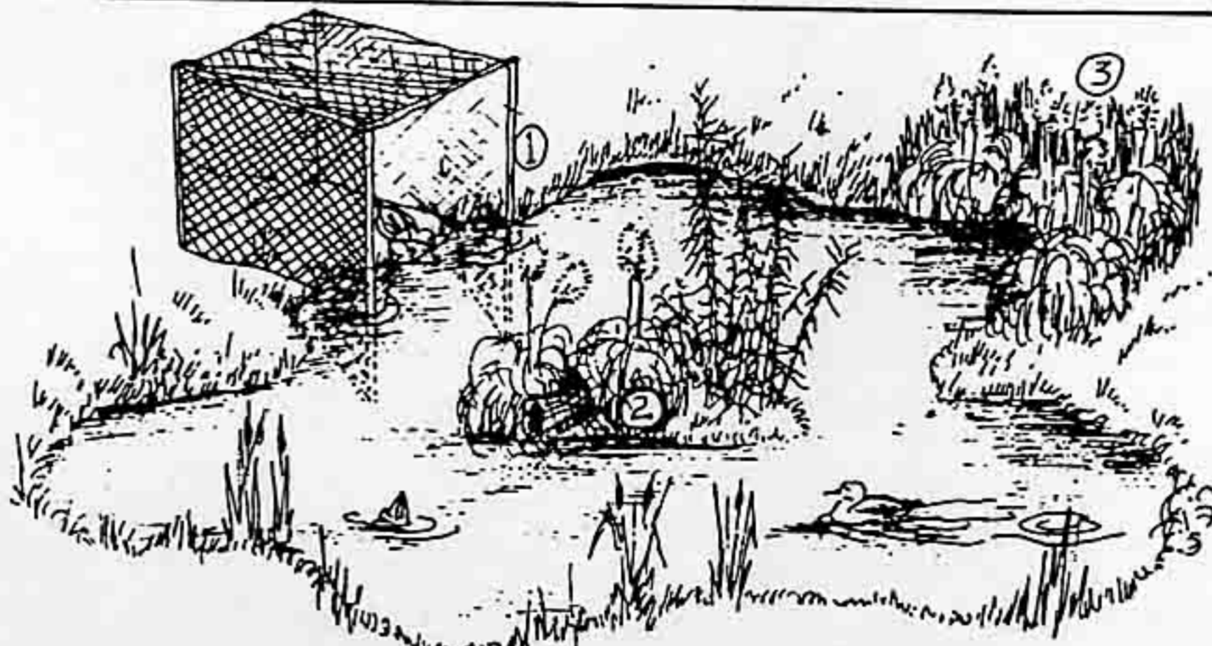
FIG. 8.4 : PROTECTION DES VOLAILLES D'EAU CONTRE LES RENARDS. 1. CAGE OUVERTE SUR L'EAU. 2. ÎLE A HERBES DES PAMPAS, BAMBOUS, BÛCHES CREUSES. 3. COIN MARÉCAGEUX, PEU PROFOND, AVEC UNE BORDURE D'HERBE DES PAMPAS.
