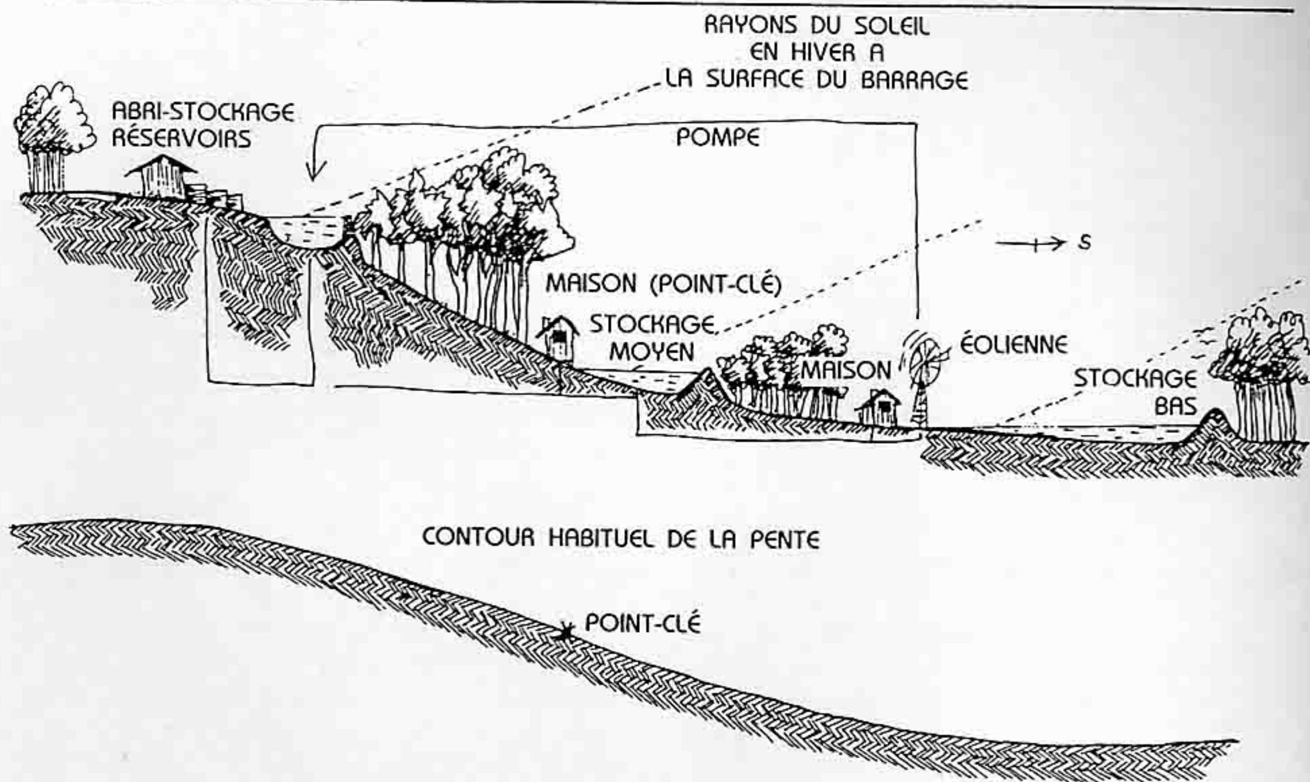
: FIG. 2.7 : EMBLACEMENT IDÉAL DES ÉLÉMENTS EN RELATION AVEC LA PENTE.
