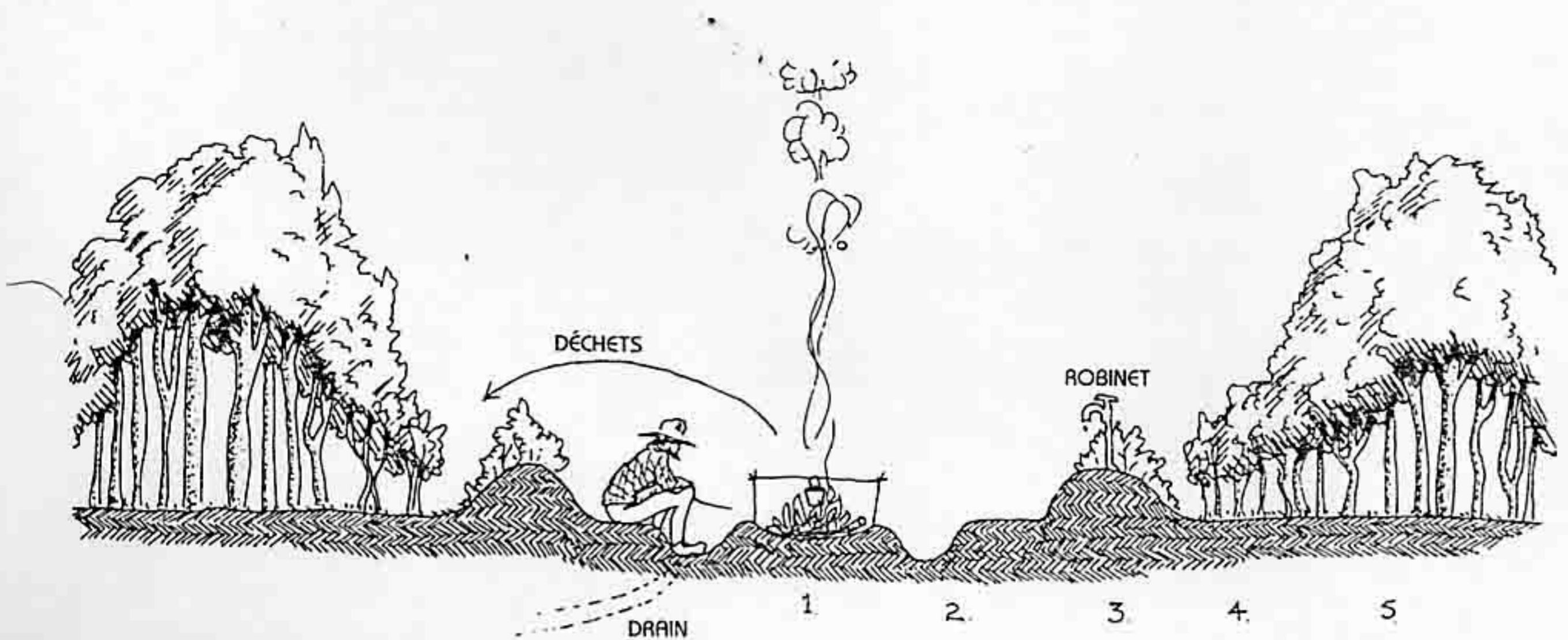
FIG. 6.18 : MANDALA DE FEU (SECTION).
