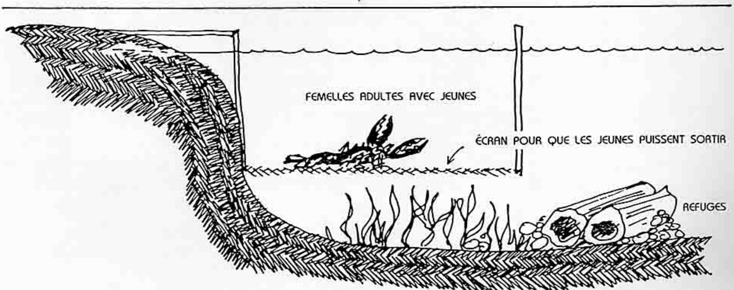
FIG. 7.19 : PANIER A FRAI POUR CRUSTACÉS D'EAU DOUCE PORTANT LEUR ŒUFS ET LEURS JEUNES SOUS LA QUEUE (ÉCREVISSSES, HOMARDS).
