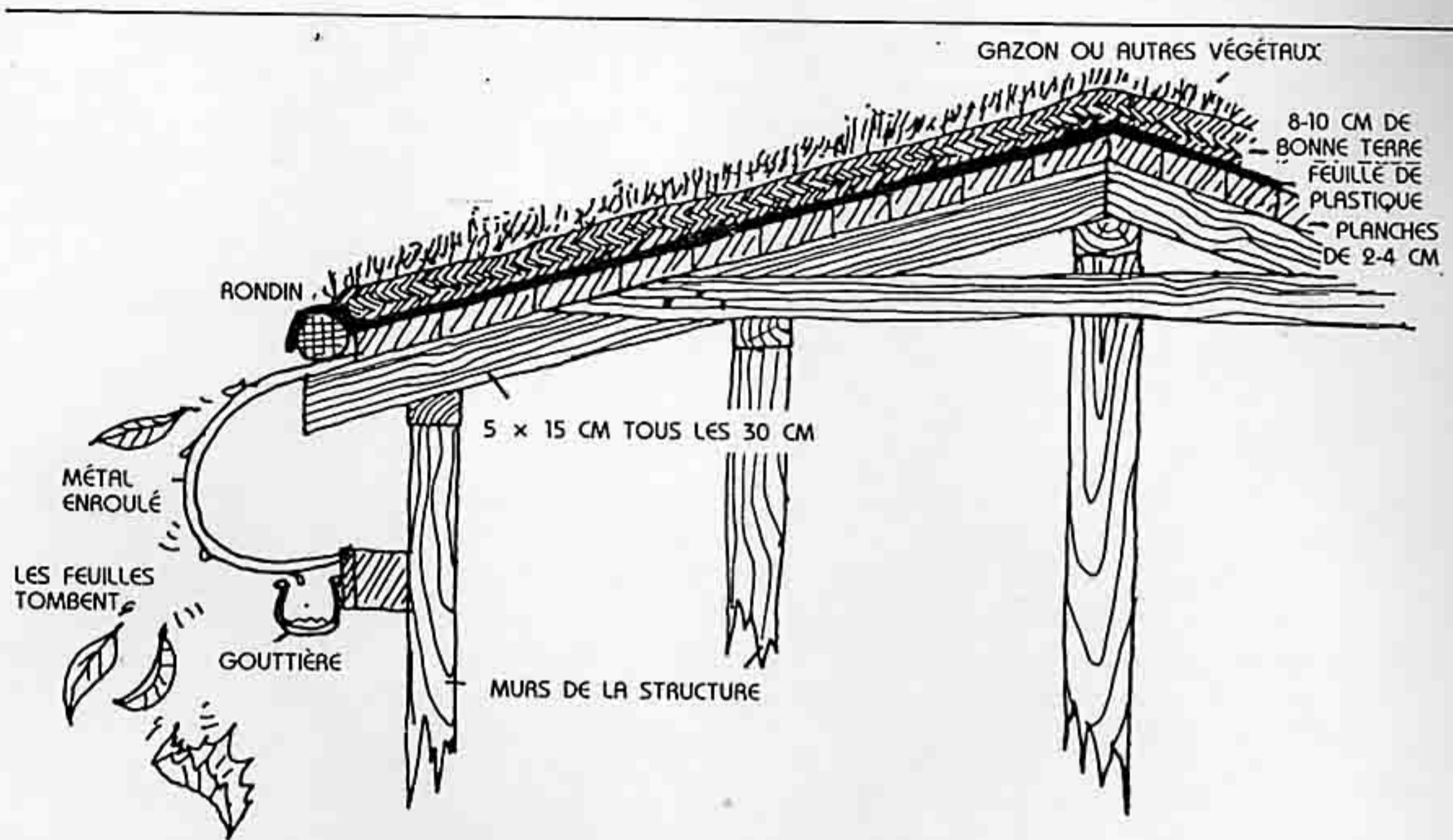
FIG. 6.16 : COUPE D'UN TOIT GAZONNÉ.
