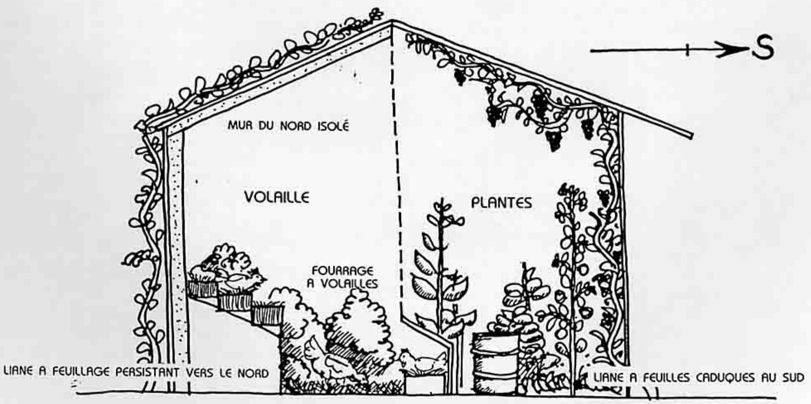
FIG. 8.3 : SERRE CHAUFFÉE PAR LES POULES.
