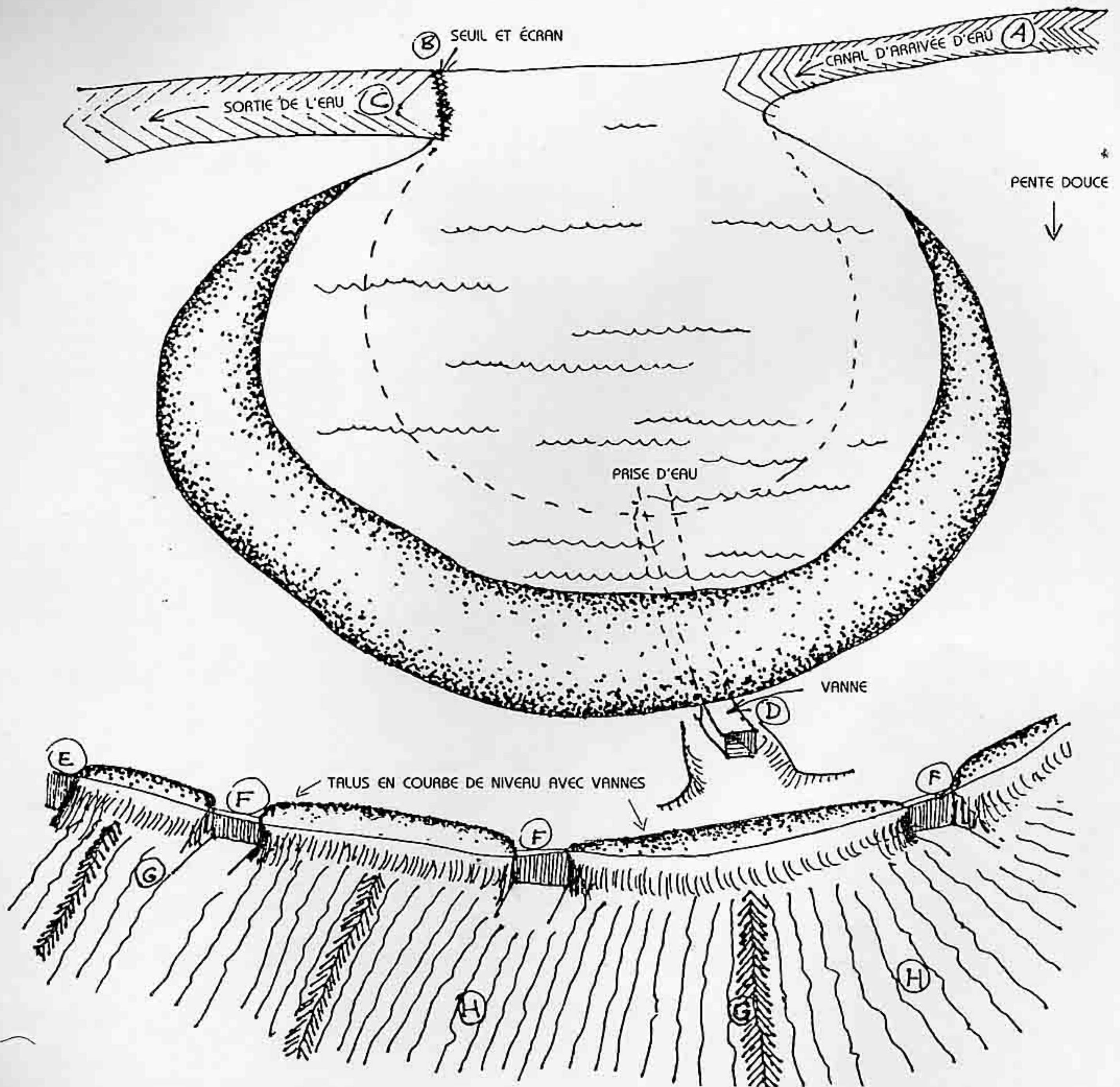
FIG. 7.14 : LA RETENUE SUPÉRIEURE RECUEILLE L'EAU VENANT DE A PAR UN CANAL (DE DÉRIVATION) COUPANT LA PENTE. EN CAS D'INONDATION, L'EAU EN EXCÈS SE DÉVERSE EN B DANS LE CANAL DE SORTIE C OU PEUT ÊTRE RELÂCHÉE A TOUT MOMENT PAR LA VANNE D. LE TALUS EN COURBE DE NIVEAU E RETIEN L'EAU LIBÉRÉE QUI PASSE DANS LES CHAMPS H SOUS LE CONTRÔLE DES VANNES F. L'EAU EST ENSUITE DIRIGÉE AU MOYEN DE LEVÉES DE TERRE TRÈS BASSES G ET S'INFILTRE DANS LES CHAMPS SOUS-SOLÉS. LA DIRECTION DU TRAVAIL DU SOL EST INDICUÉE PAR LES LIGNES ESPACÉES (D'APRÈS LE BARRAGE CONÇU A DIGGER'S REST PAR KEN YEOMANS).
