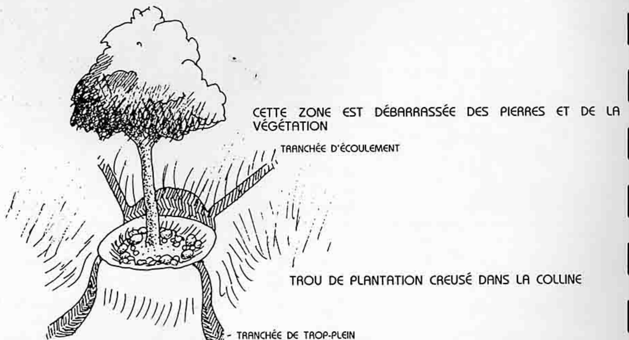
FIG. 5.4 : DÉTAIL D'UNE CUVETTE.
