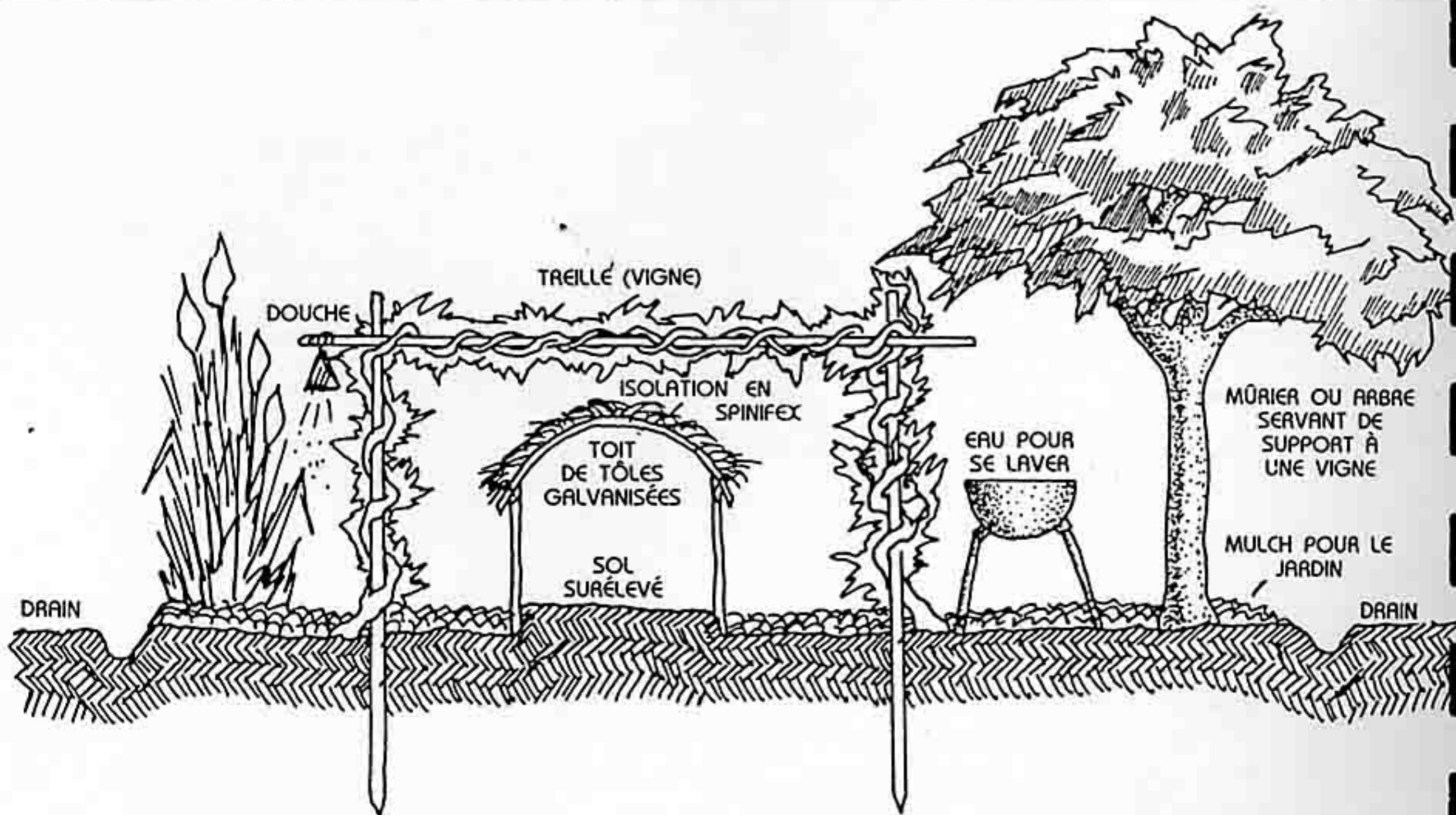
FIG. 5.1 : SECTION D'UNE WILTJA IDÉALE.
