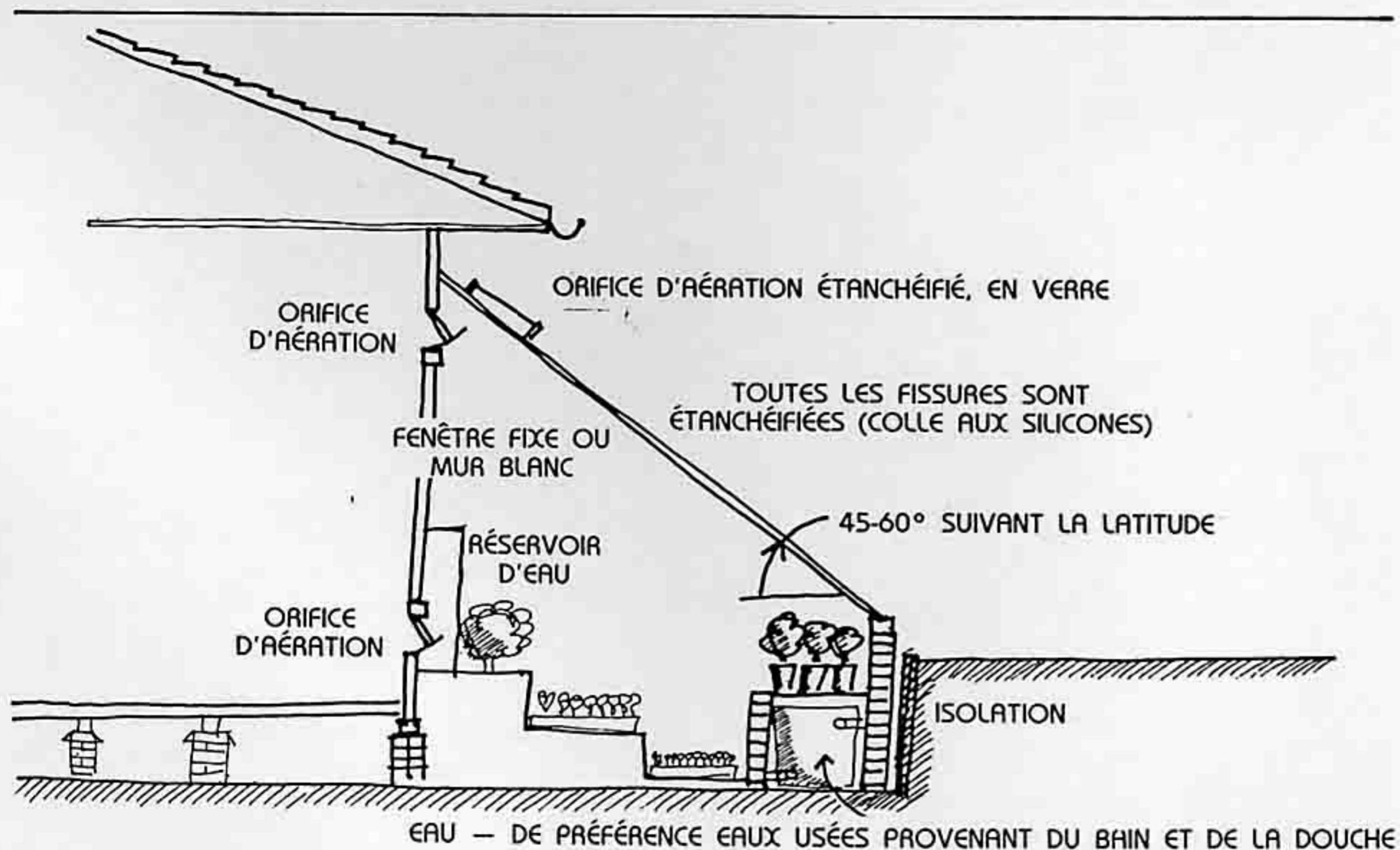
FIG. 6.3 : POINTS PRINCIPAUX DE LA SERRE INTÉGRÉE.
