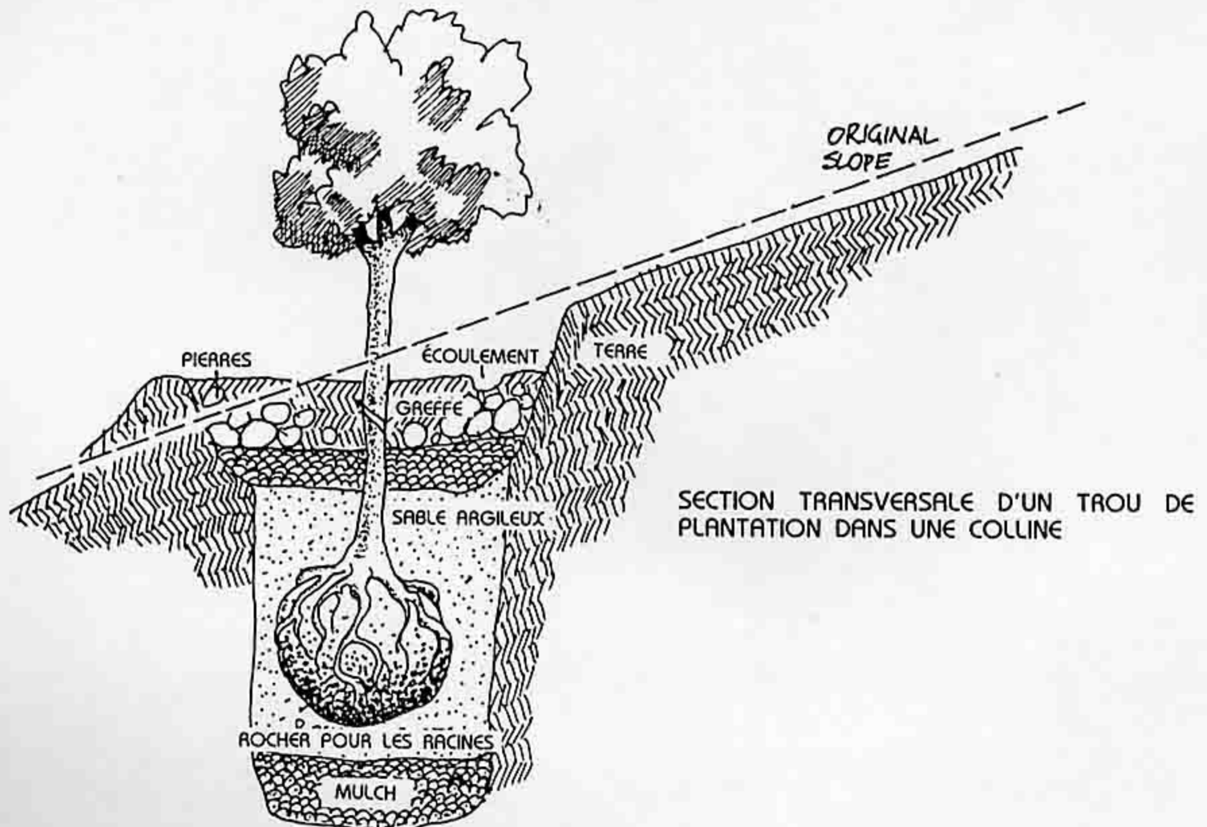
FIG. 5.18 : DÉTAIL D'UN TROU DE PLANTATION.
