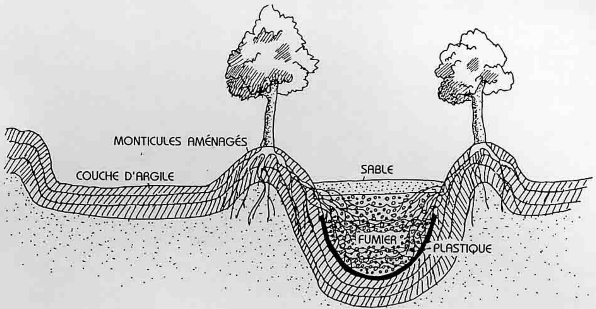
FIG. 5.16 : DES « Puits » de fumier dans des couches d'argile stockent les eaux d'inondation pour les plantes sur les monticules.
