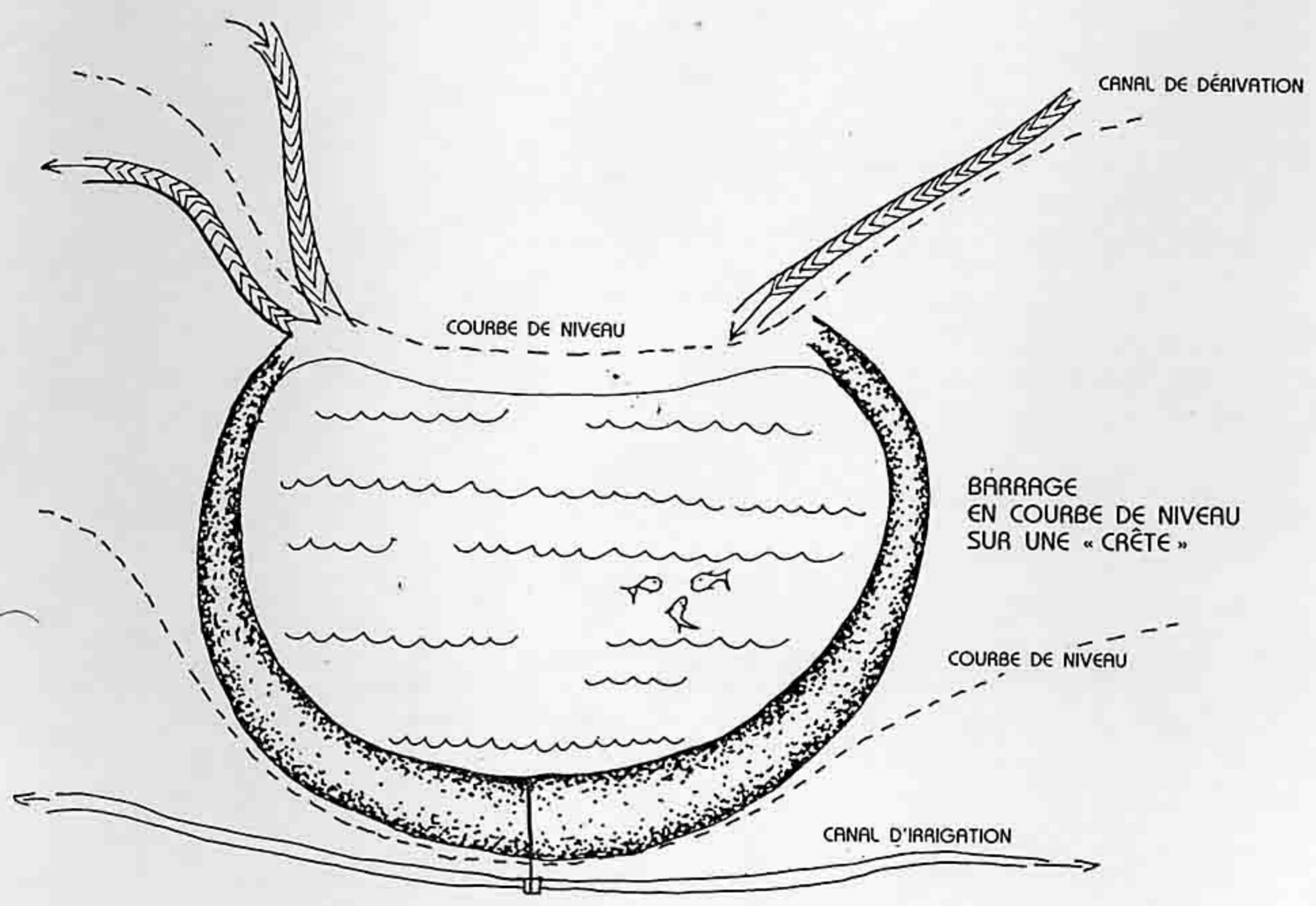
FIG. 7.4 : BARRAGES EN COURBES DE NIVEAU.
