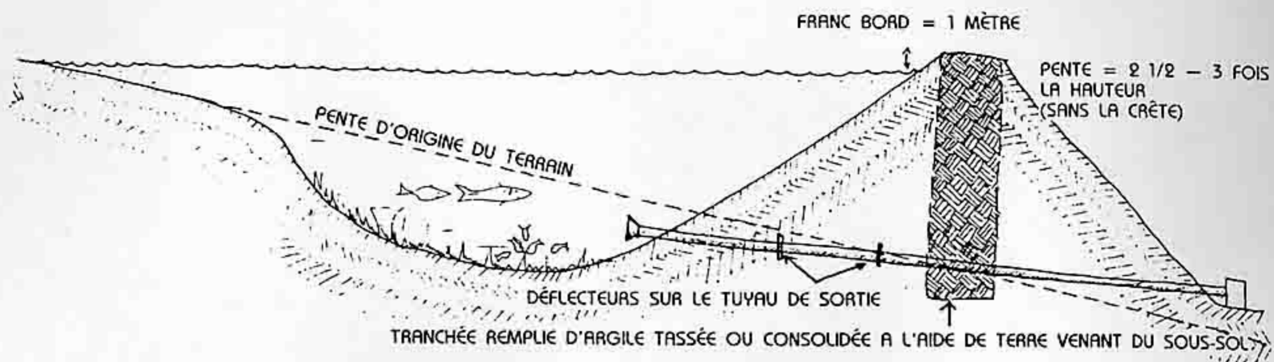
FIG. 7.2 : UN BARRAGE CLASSIQUE (D'APRÈS YEOMANS ® ). SECTION.
