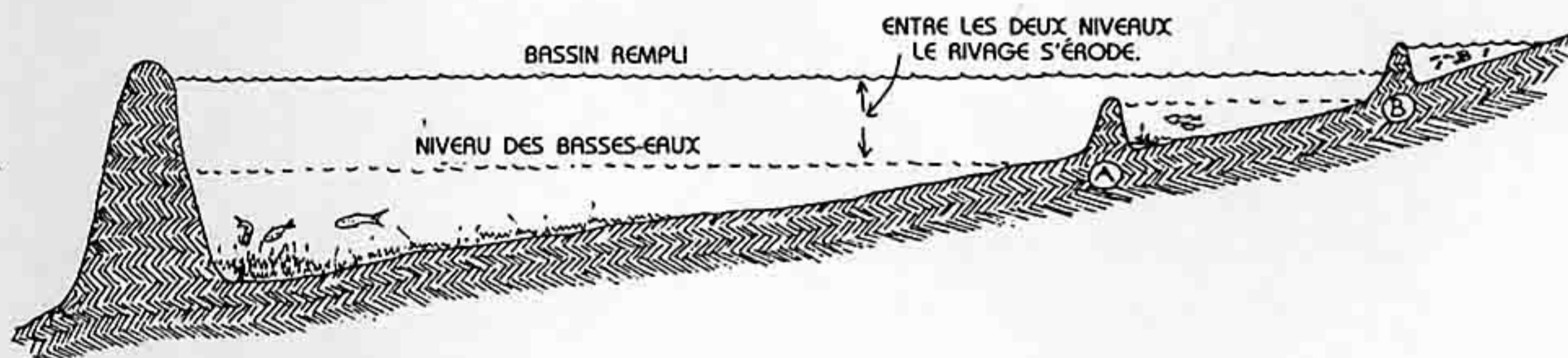
FIG. 7.8 : MODIFICATIONS DU CAPTAGE PRINCIPAL (SECTION).
