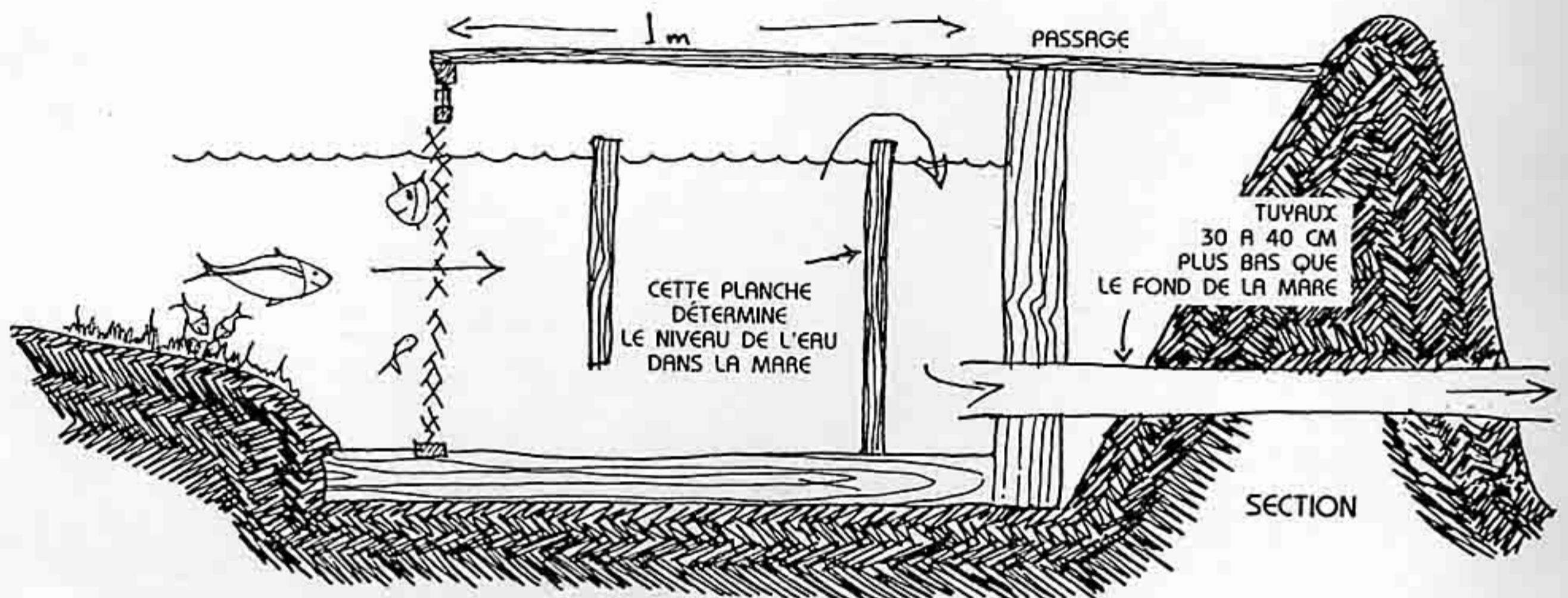
FIG. 7.15 : L'ÉCRAN A POISSONS CLASSIQUE « HERGUTH MONK », AVEC TROP-PLEIN POUR ÉCOULEMENT CONSTANT.
