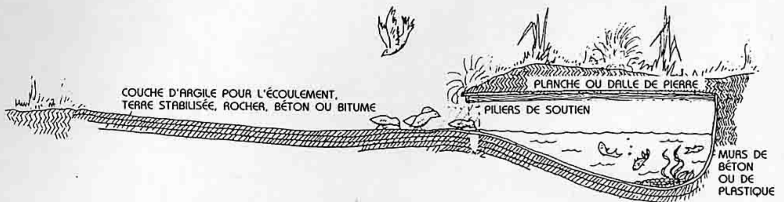
FIG. 5.14 : UN PETIT Puits DANS UNE COUCHE D'ARGILE OU A LA BASE D'UN ROCHER RETIEN L'EAU POUR CAILLES, PIGEONS, LÉZARDS ET ABEILLES. POISSONS ET MOULES MAINTIENNENT L'EAU CLAIRE. LE BÉTAIL NE PEUT SALIR DE TELS Puits.
