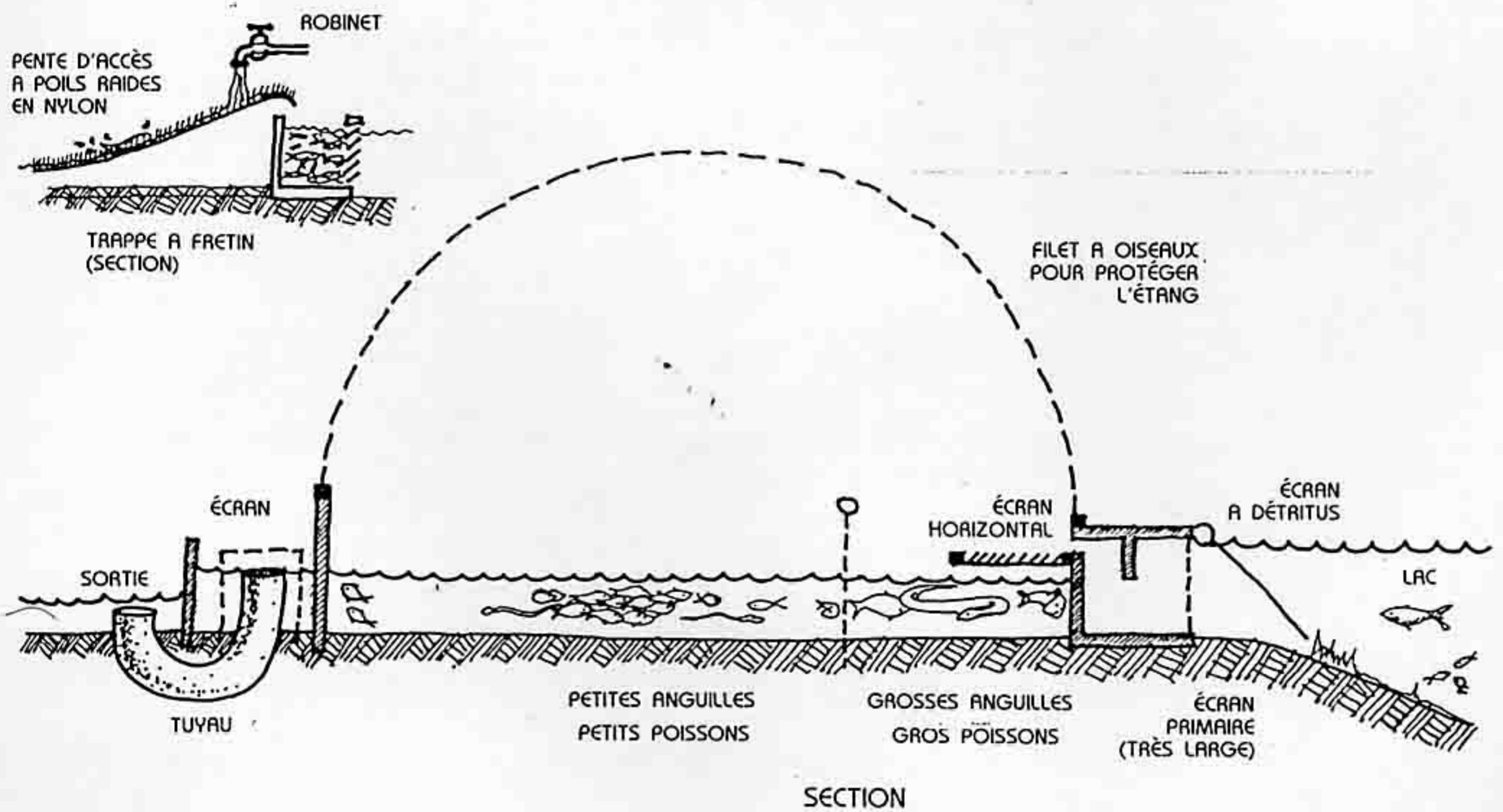
FIG. 7.23 : SORTIE COMPLEXE POUR LA CAPTURE EN AMONT DE FRETIN ET DE CIVELLES, EN AVAL D'ADULTES (ANGUILLES ET AUTRES POISSONS). L'ÉTANG RETIENT LES ADULTES DESCENDANT VERS LA MER.
