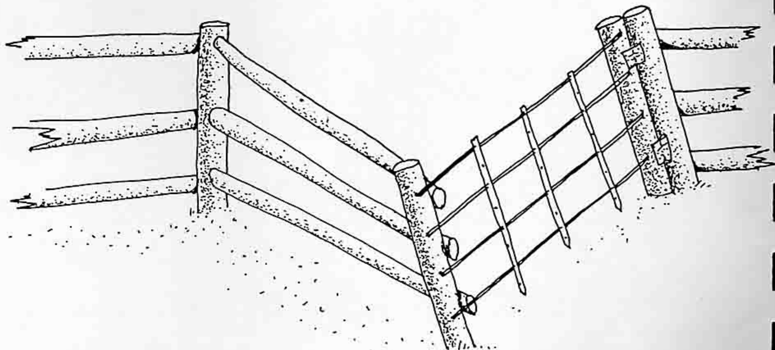
FIG. 5.23 : DÉTAIL DE LA PORTE DE L'ENCLOS-PIÈGE. LES POTEAUX INCLINÉS FONT QUE LA PORTE D'ACIER RETOMBE ET SE FERME APRÈS QUE LES BOVINS ET LES CHEVAUX L'ONT OUVERTE POUR ACCÉDER À L'EAU (L'INCLINAISON EST EXAGÉRÉE ICI). D'APRÈS LE PIÈGE DE WARRENS CREEK.
