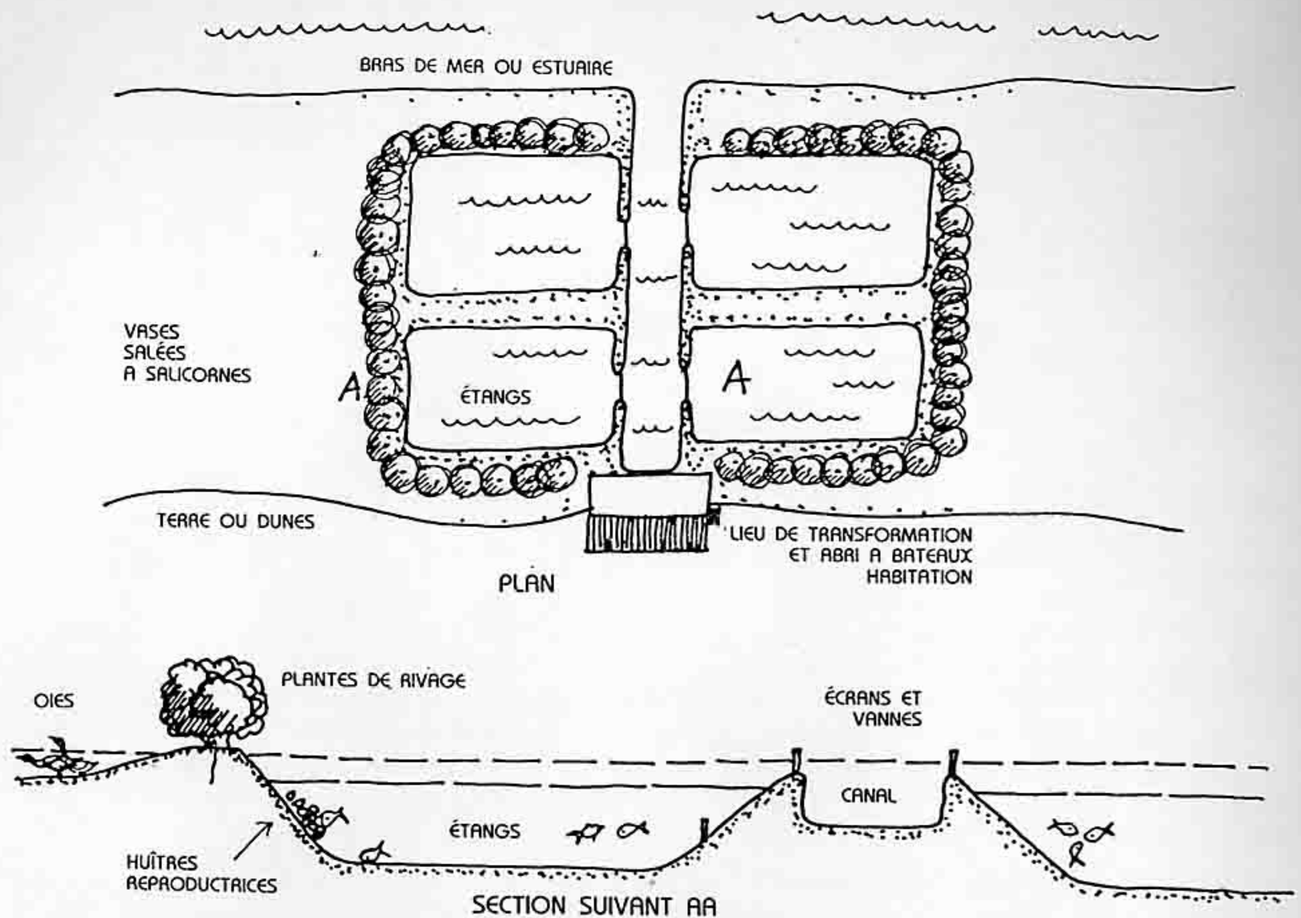
FIG. 7.24 : PLAN ET SECTION D'ÉTANGS A MARÉE.
