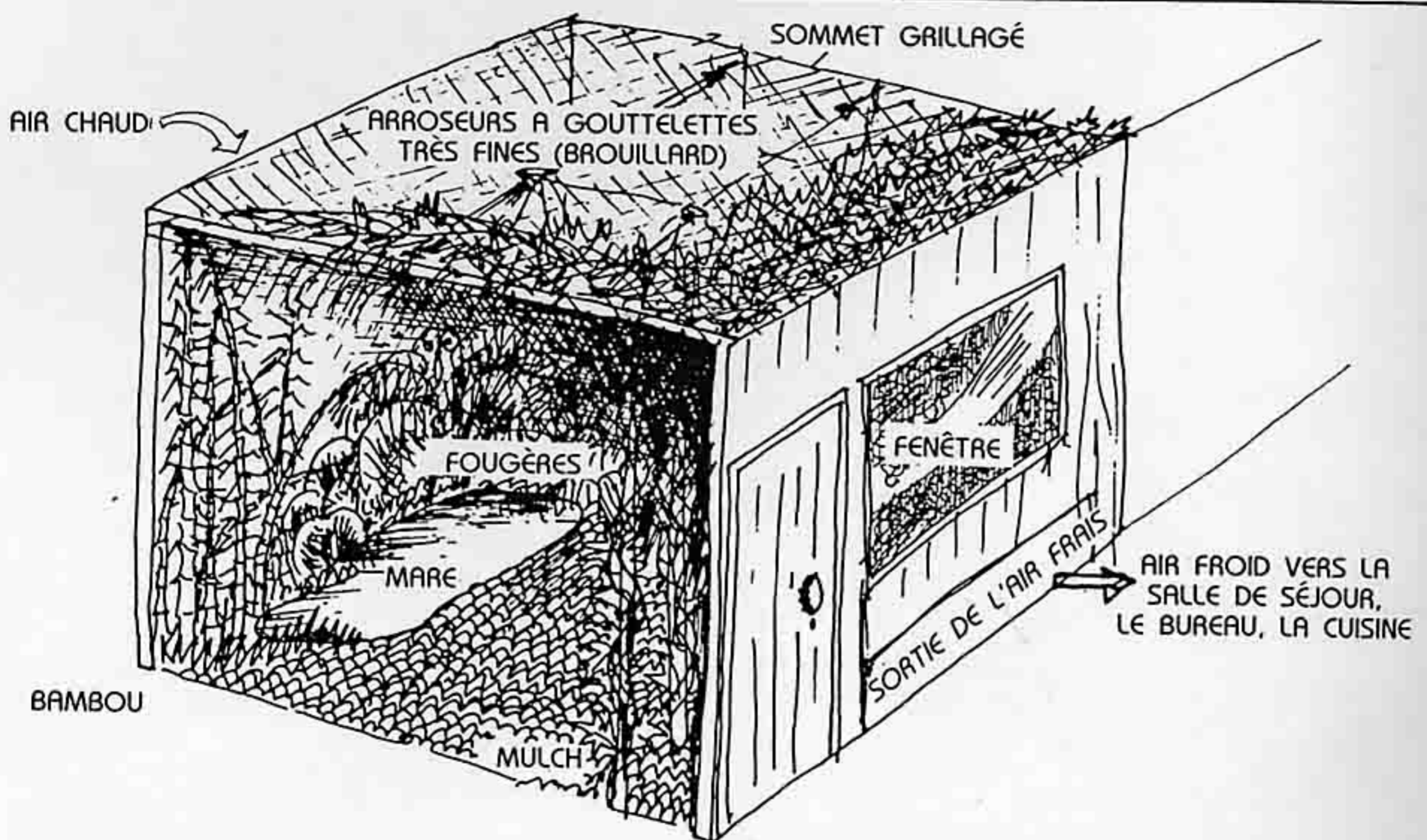
FIG. 6.4 : « MAISON D'OMBRE » AU NORD DE LA CUISINE, DU BUREAU, DE LA BUANDERIE, DU COULOIR D'ENTRÉE.
